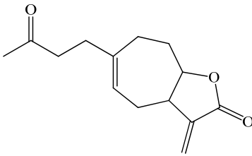
xanthinosin
