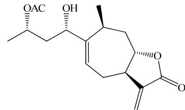
xanthanol
