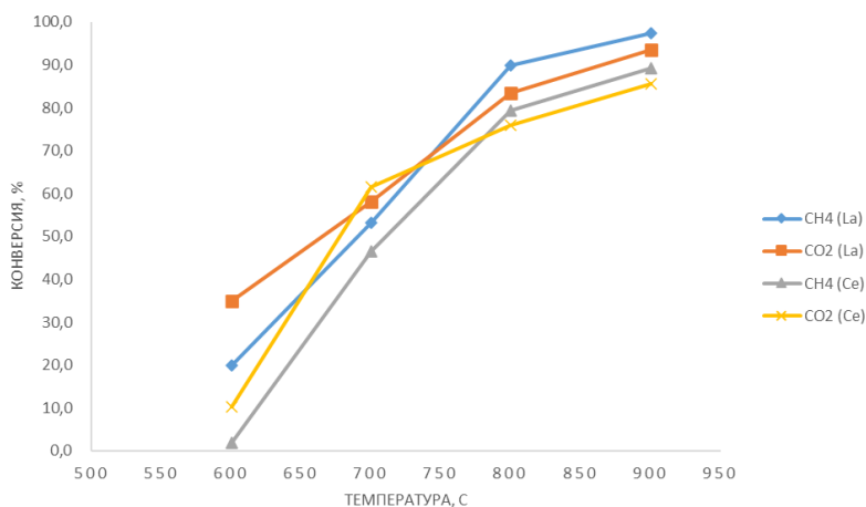
Рисунок 1 - Зависимость конверсии метана и \text{CO}_2 от температуры реакции на катализаторах Co-La-Al и Co-Ce-Al
