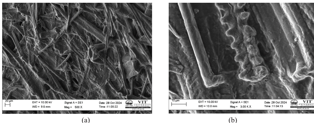
Сурет 1. Арпа сабағына алынған целлюлоза мен хитозан негізіндегі глицерин арқылы алынған үлгі: (a) АЦХПЭГ-1 (хитозан мөлшері 1%), (b) АЦХПЭГ-3 (хитозан мөлшері 3%)
