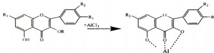
Сурет 1 - Флавоноидтардың алюминий хлоридімен комплекс түзілу реакциясы
