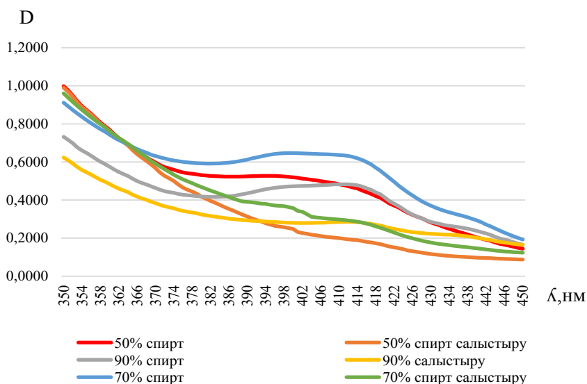
Сурет 3 - Флавоноид пен алюминий хлориді комплекстерінің әртүрлі экстрагенттердегі спектрлері
