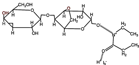
Рисунок 3. Схема взаимодействия агар-агар, ПЭОЗ и I_2/KI
