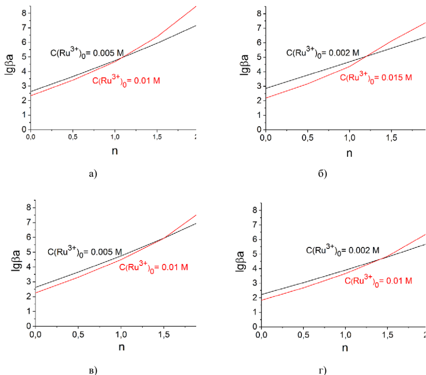
Рисунок 1. Зависимость между \lg \beta_a и n при взаимодействии: (а) полиакриламида (0,01 М) с \text{Ru}^{3+} (0,005 и 0,01 М), (б) полиакриловой кислоты (0,015 М) с \text{Ru}^{3+} (0,002 и 0,015 М), (в) хитозана (0,01 М) с \text{Ru}^{3+} (0,005 и 0,01 М) и (г) поли-4-винилпиридина (0,025 М) с \text{Ru}^{3+} (0,002 и 0,01 М)
